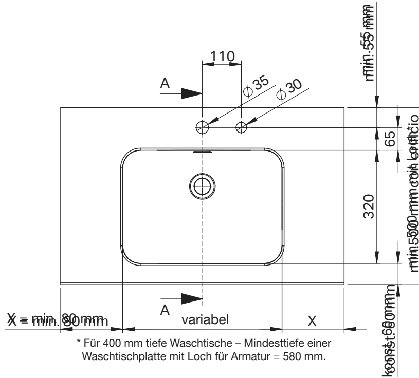
DRAUFSICHT
